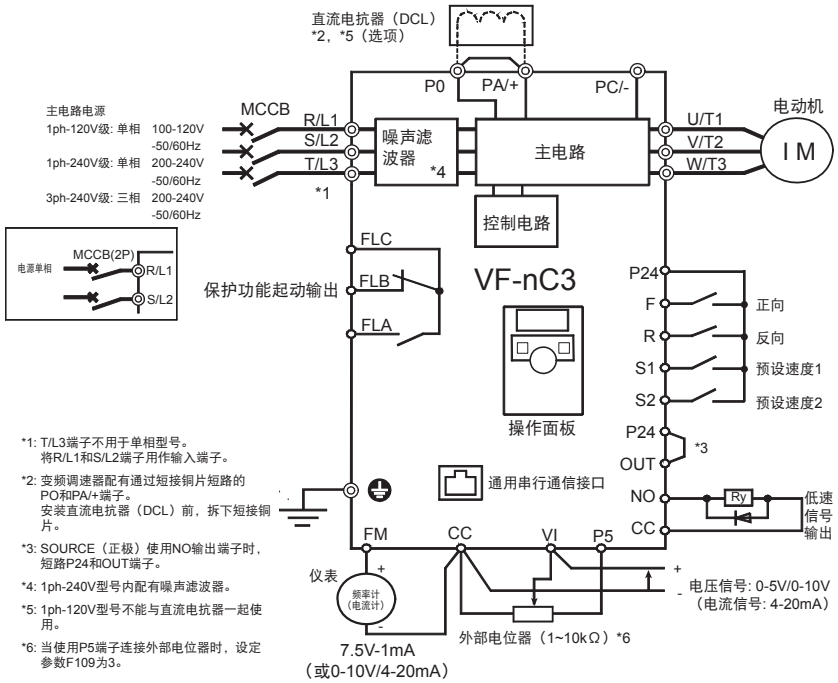
标准连接图-SOURCE（正极）（通用: P24）
